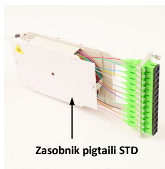
Zasobnik pigtaili STD - zabezpieczenie pigtaili w tylnej części modułu
