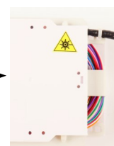
Zasobnik pigtaili STD - zabezpieczenie pigtaili w tylnej części modułu
